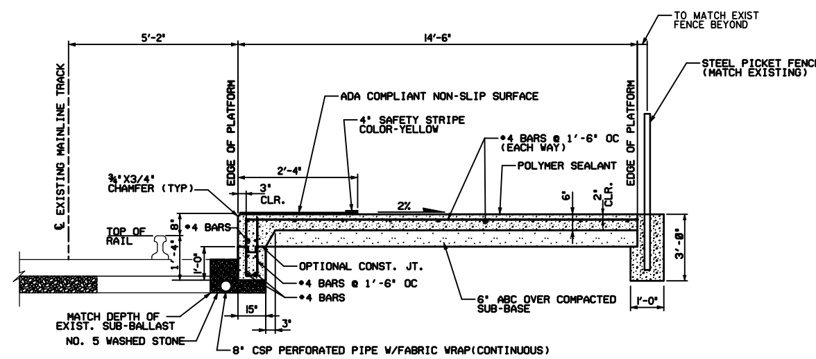
DETAIL - SECTION A-A N.T.S.
